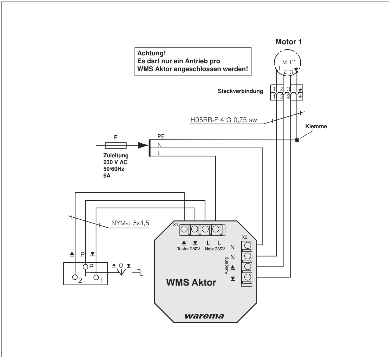
Abb. 2 Anschluss des WMS Aktors
